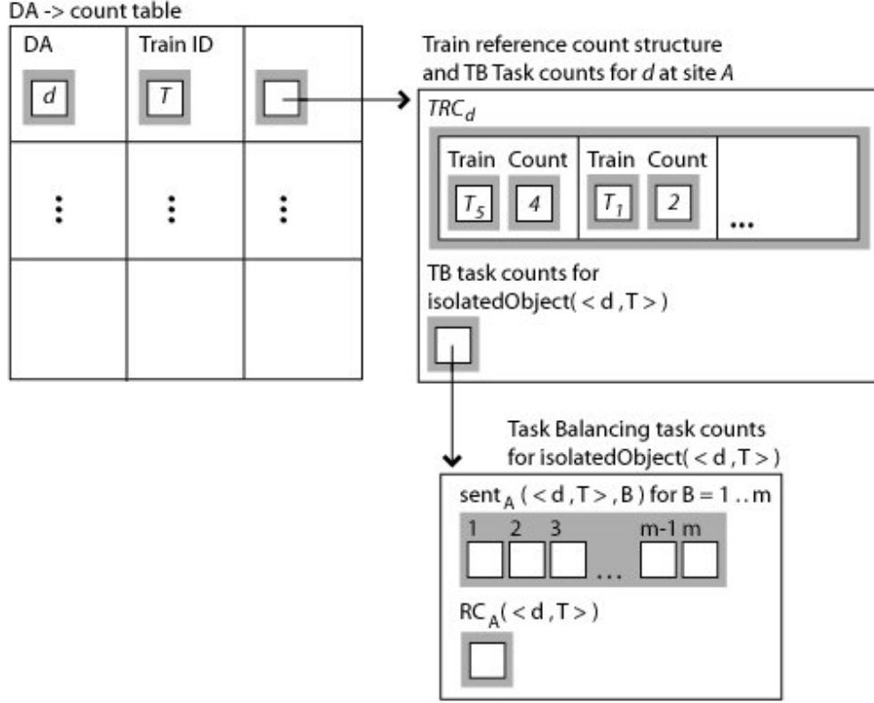
Figure 7.4 - The DA → Count Table
